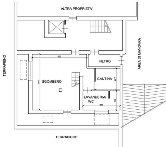
PIANTA PIANO INTERRATO
