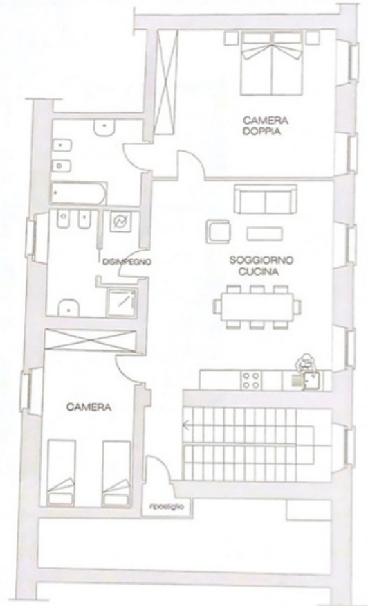
ALLOGGIO V18 - PIANO PRIMO -
